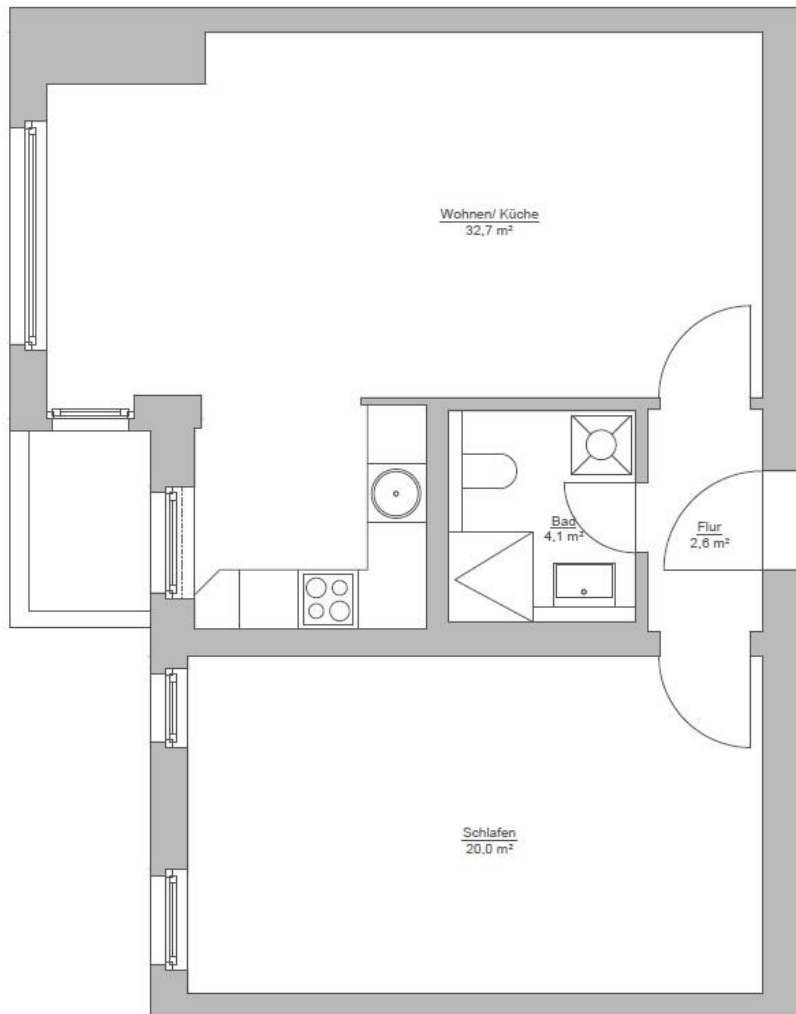
Grundriss
